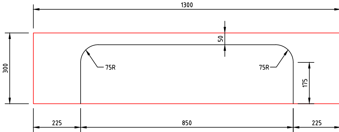
ELEVATION
